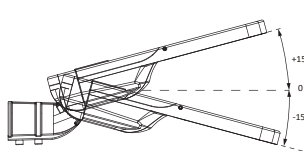
Instalación Horizontal ±0-5-10-15°
